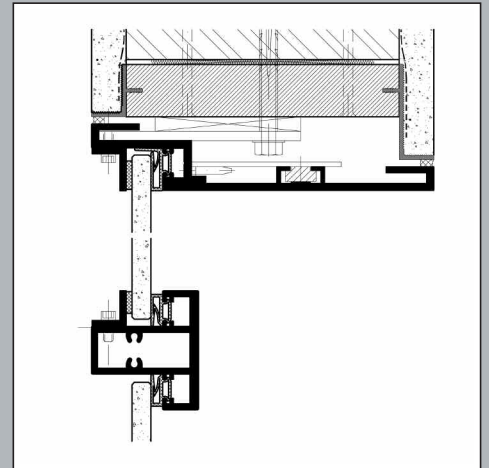
FZF slimline mit Normfalz, Ganzglastür und Kämpfer KLF für Oberlicht in Massivwand
