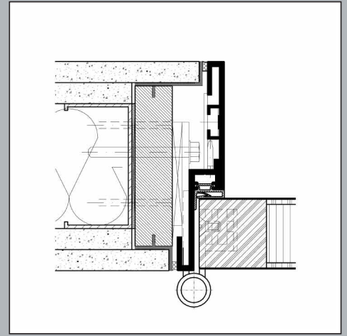
FZS slimline mit Grundzarge und Alu-Abschlussprofil in leichter Trennwand
