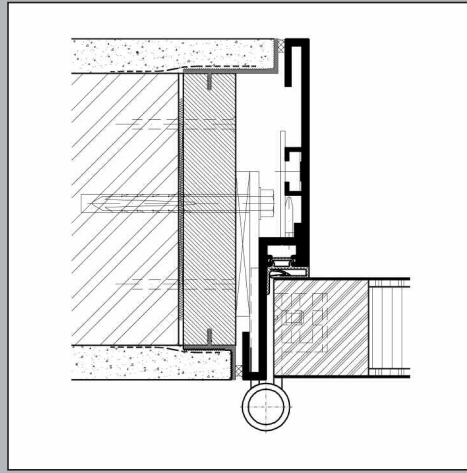
FZS slimline mit Grundzarge und Alu-Putzprofil in Massivwand
