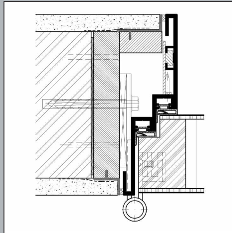
FZDS slimline in Massivwand für Schallschutzfunktion R_{w,P} 42 dB
