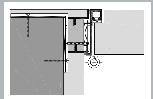
LZB slimline in Massivwand
