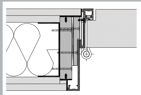
LZBS slimline mit Leibungsverkleidung in Leichtbauwand
